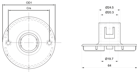
NẮP ĐẬY CÓ LỖ CHỈ DÀNH CHO ỐNG LUỒN ĐÀN HỒI Ø 20MM /uPVC JUNCTION BOX COVER USED FOR CORRUGATED CONDUIT Ø 20MM
